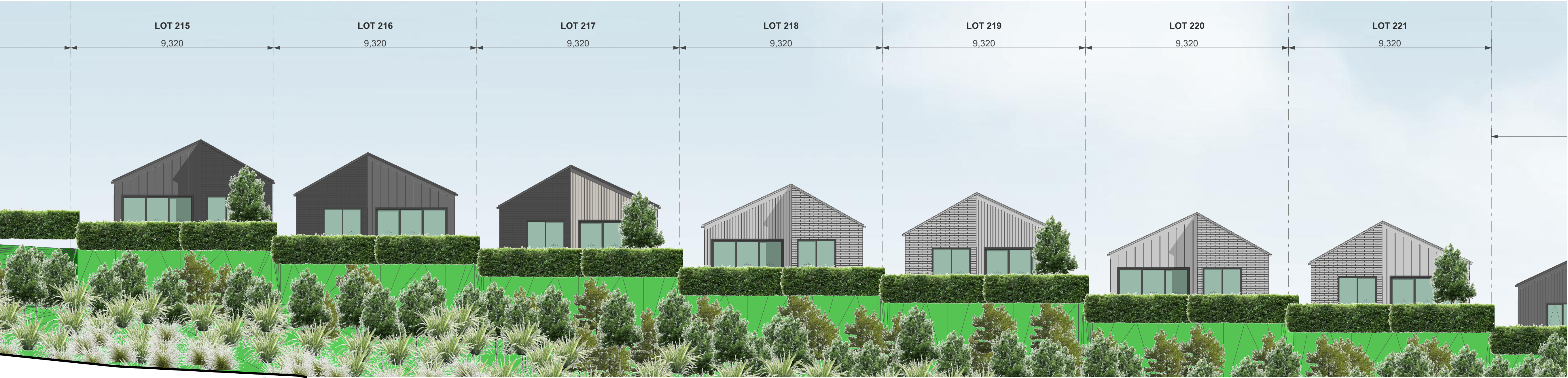
4 ELEVATION - STAGE 1A-4 - STREAM EDGE 1:100
