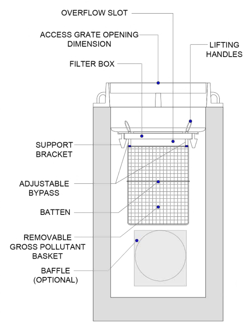
SECTION A-A
