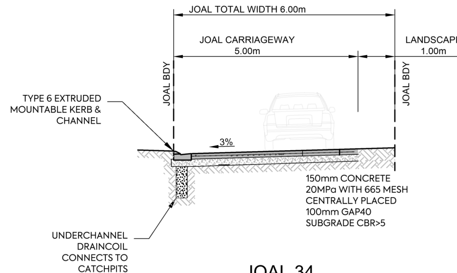
JOAL 34 F 6.0m JOAL 300 SCALE 1:100 @A3
