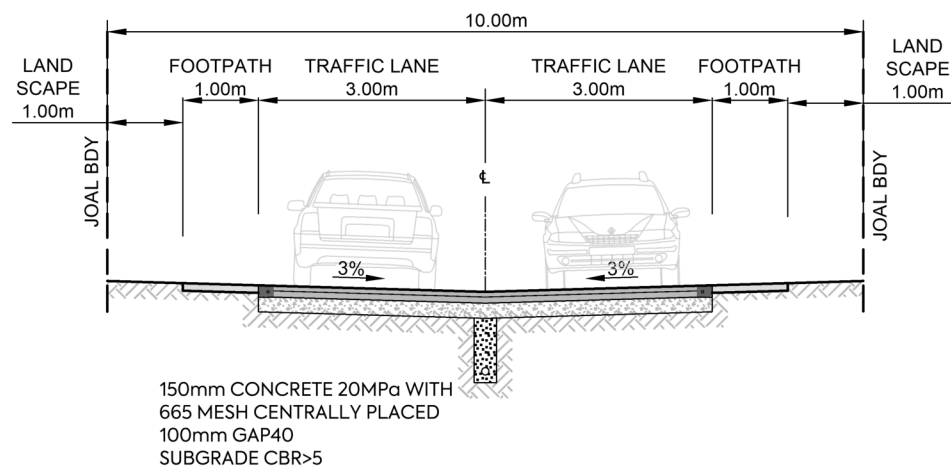
JOAL 3A, 12, 13 N1 300 10m JOAL SCALE 1:100 @A3
