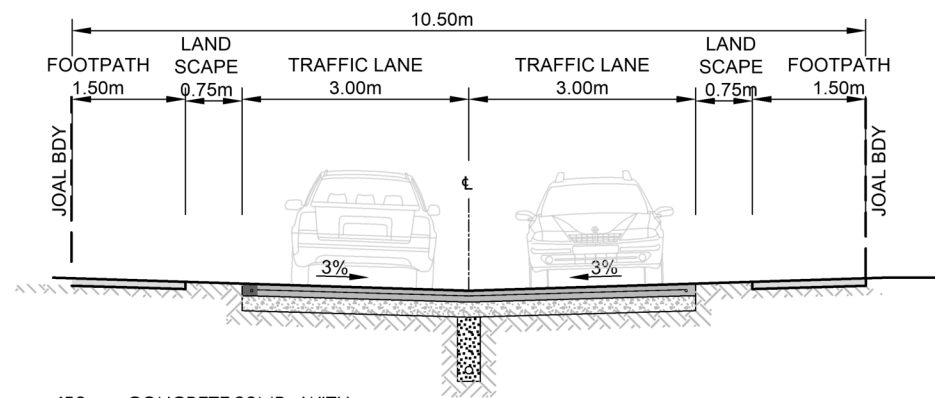
JOAL 36 10.5m JOAL SCALE 1:100 @A3
