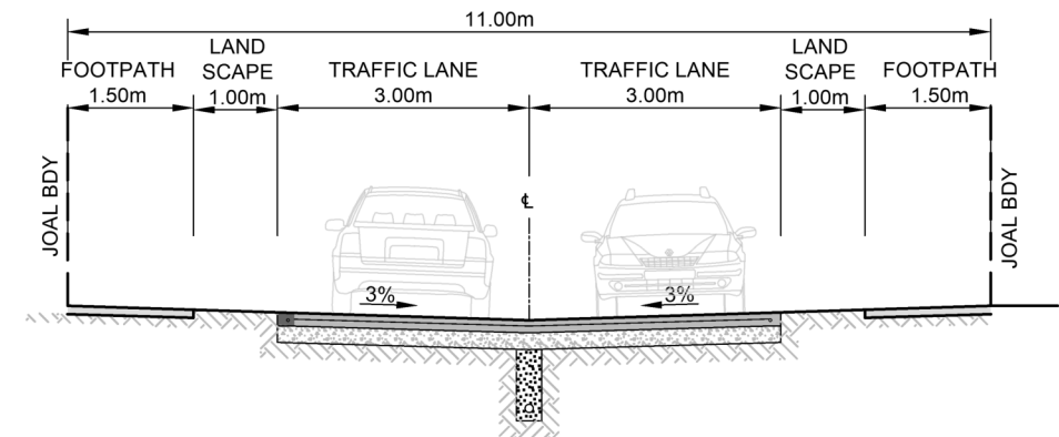
JOAL 4A, 11.0m JOAL SCALE 1:100 @A3
