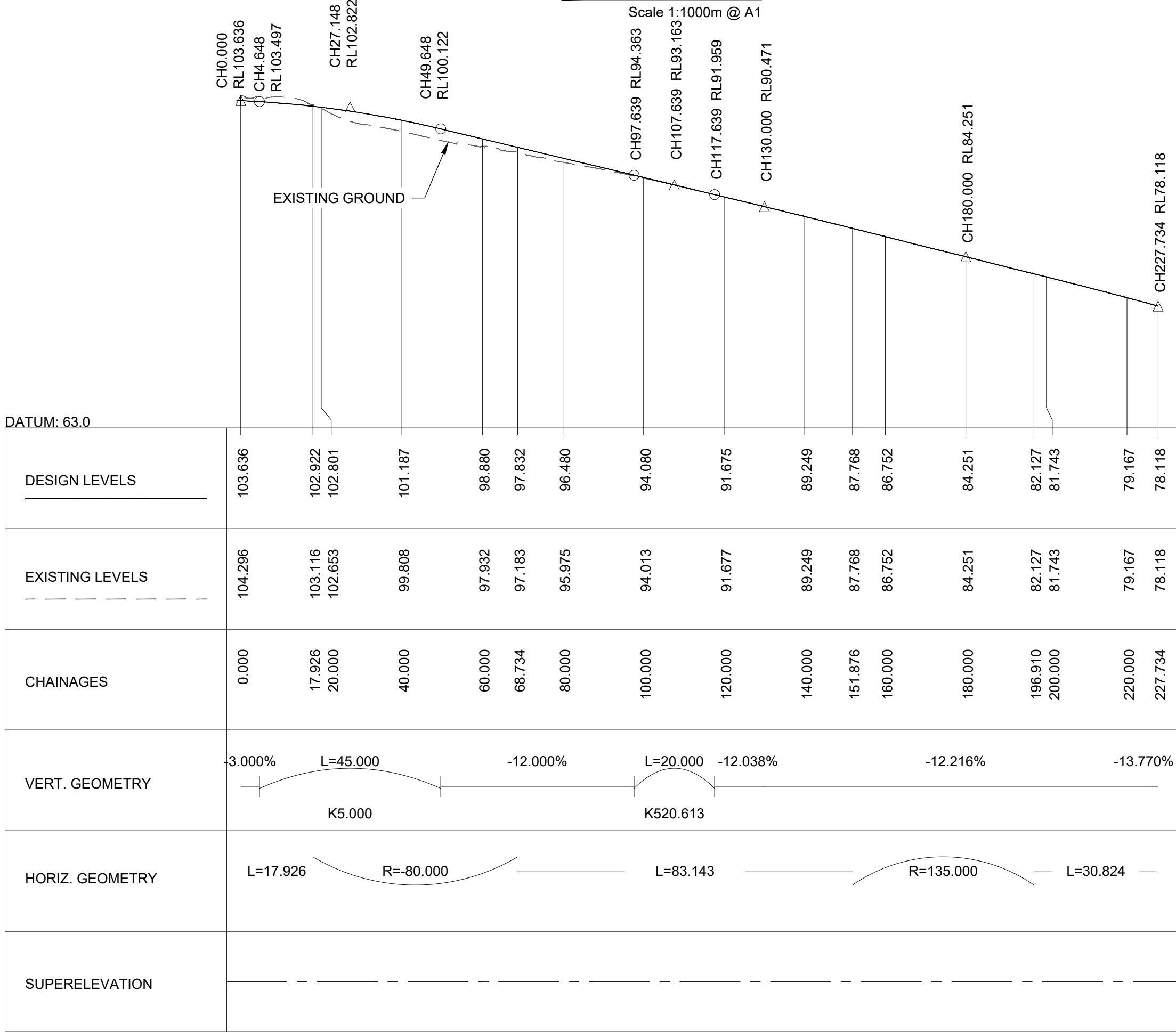
LONGITUDINAL SECTION - MC1H01
