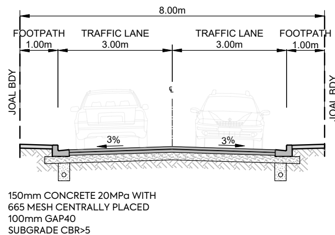
JOAL 13 8m JOAL SCALE 1:100 @A3
