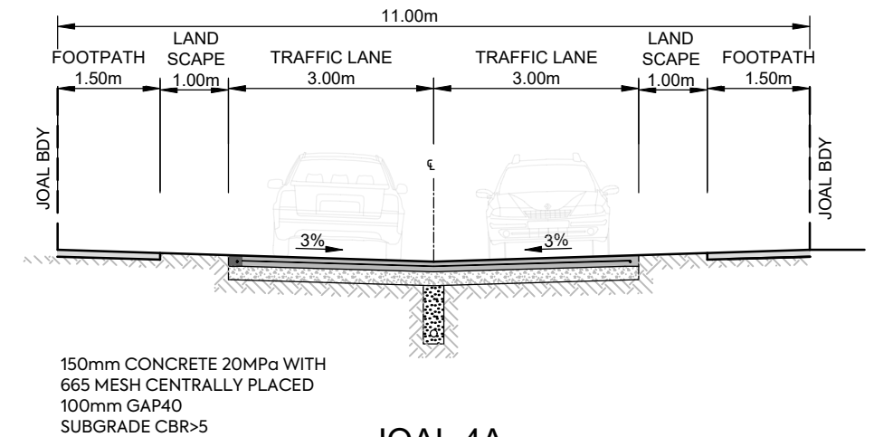
JOAL 4A, 11.0m JOAL SCALE 1:100 @A3
