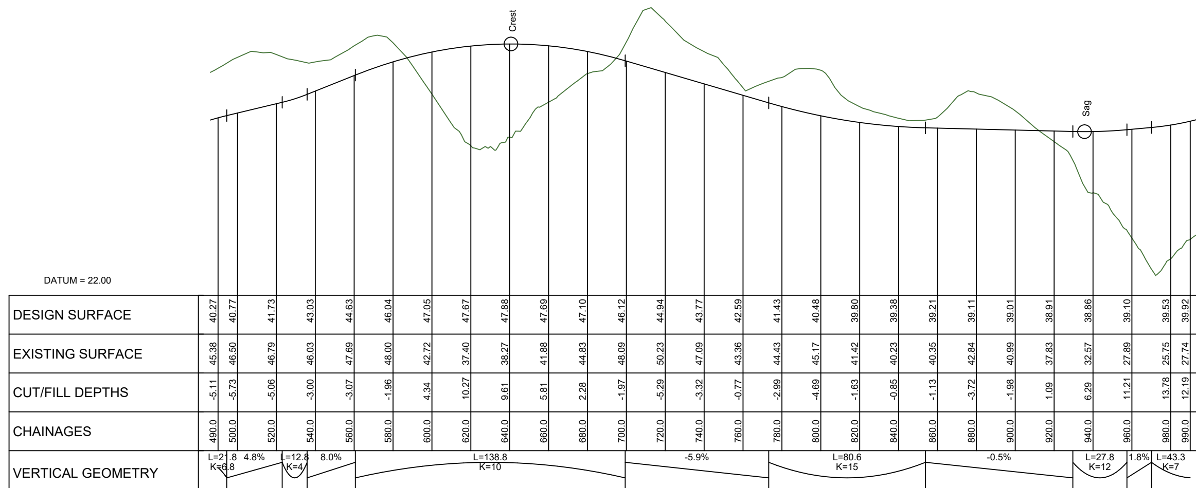
LONGITUDINAL SECTION NOR 6
