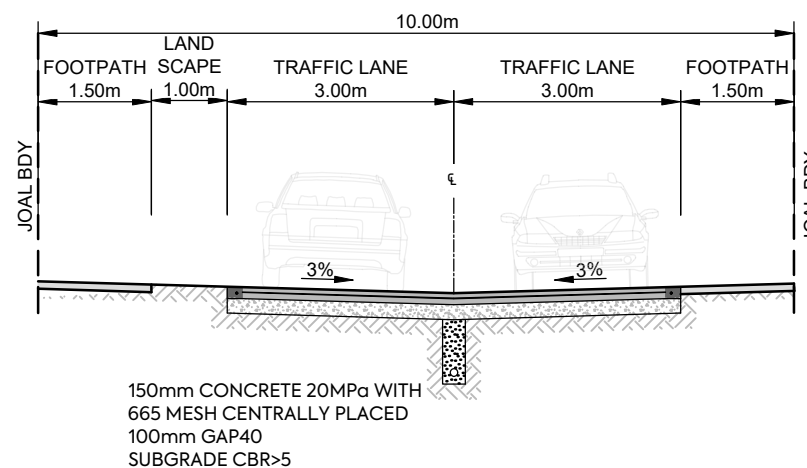
JOAL 3, 3a, 9 10m JOAL SCALE 1:100 @A3
