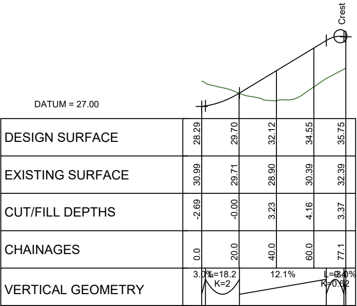
LONGITUDINAL SECTION JOAL30 SCALE HORIZ=1:2000 @ A1 VERT=1:400 @ A1
