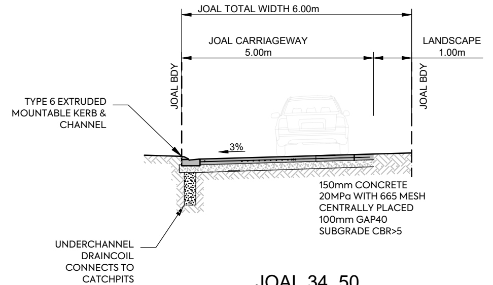
JOAL 34, 50 6.0m JOAL SCALE 1:100 @A3
