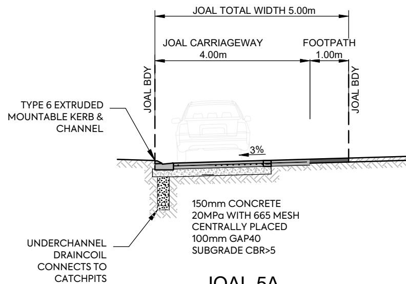
JOAL 5A 5.0m JOAL SCALE 1:100 @A3
