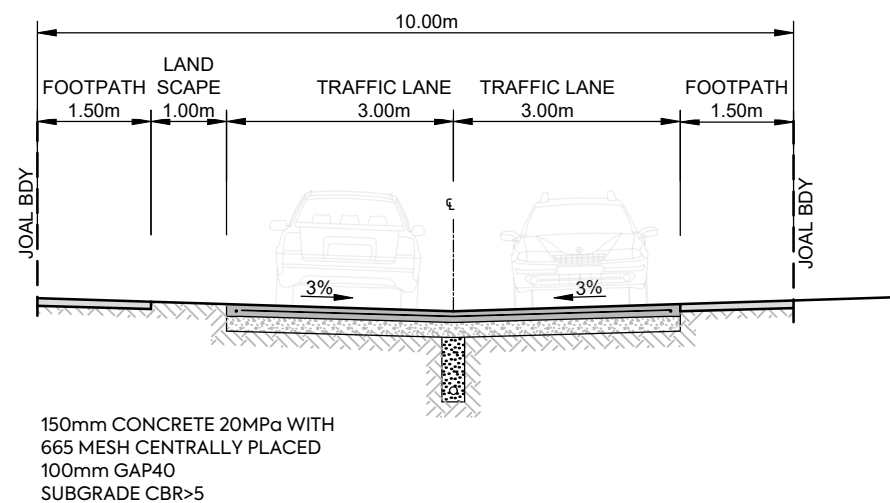
JOAL 1 10m JOAL SCALE 1:100 @A3
