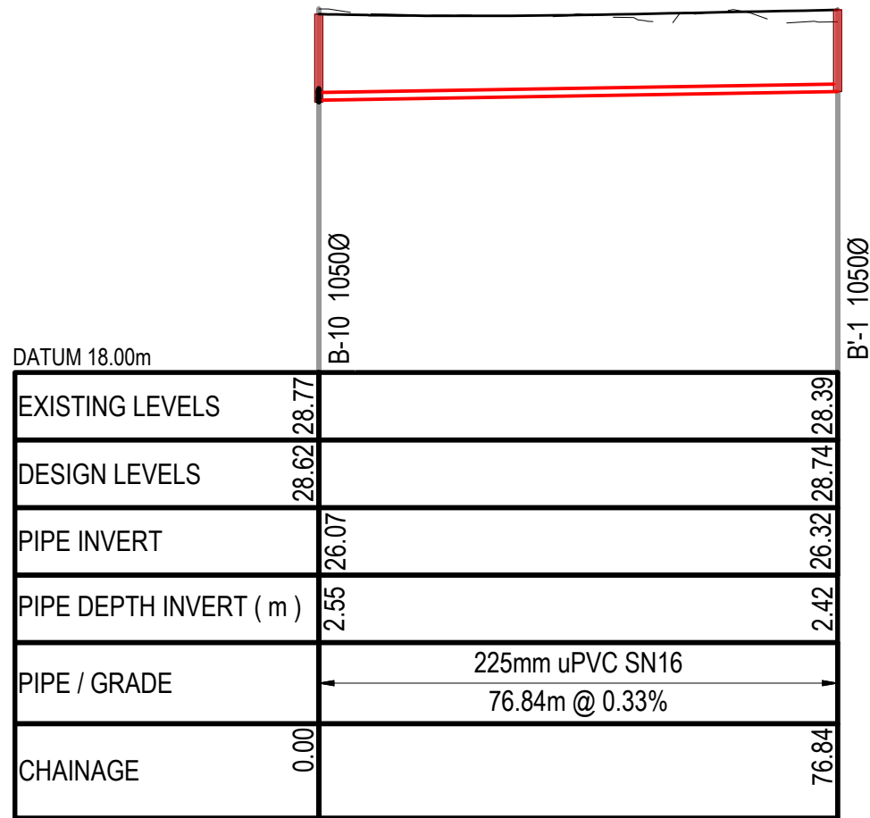
WASTEWATER LINE B' SCALE: HORI 1:1000 VERT 1:200
