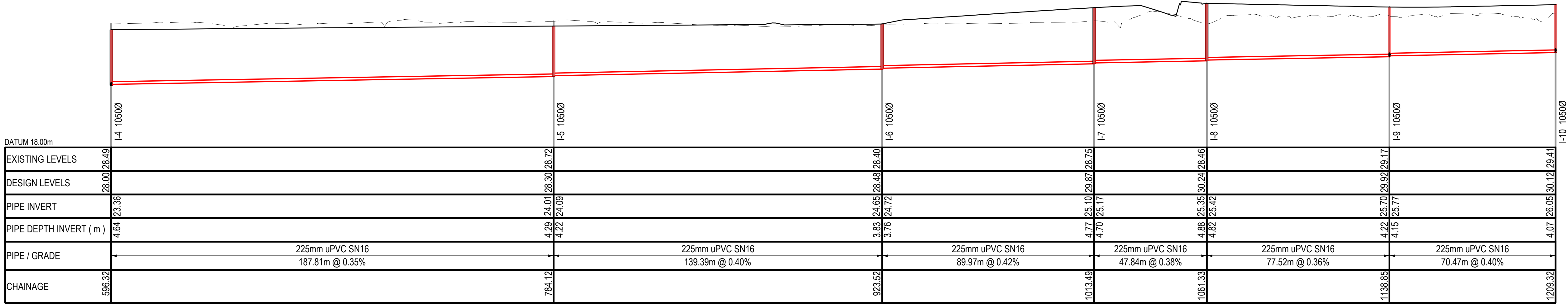
WASTEWATER LINE I SCALE: HORI 1:1000 VERT 1:200
