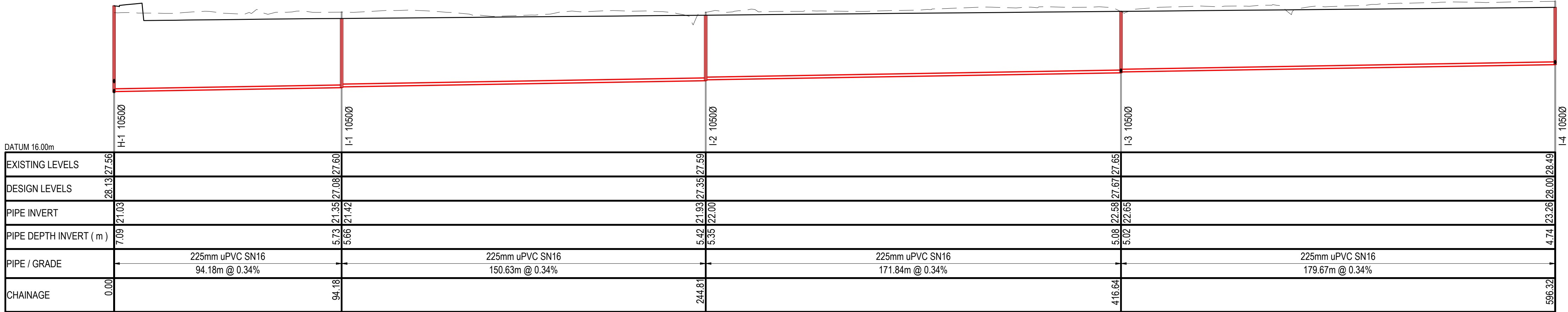
WASTEWATER LINE I SCALE: HORI 1:1000 VERT 1:200
