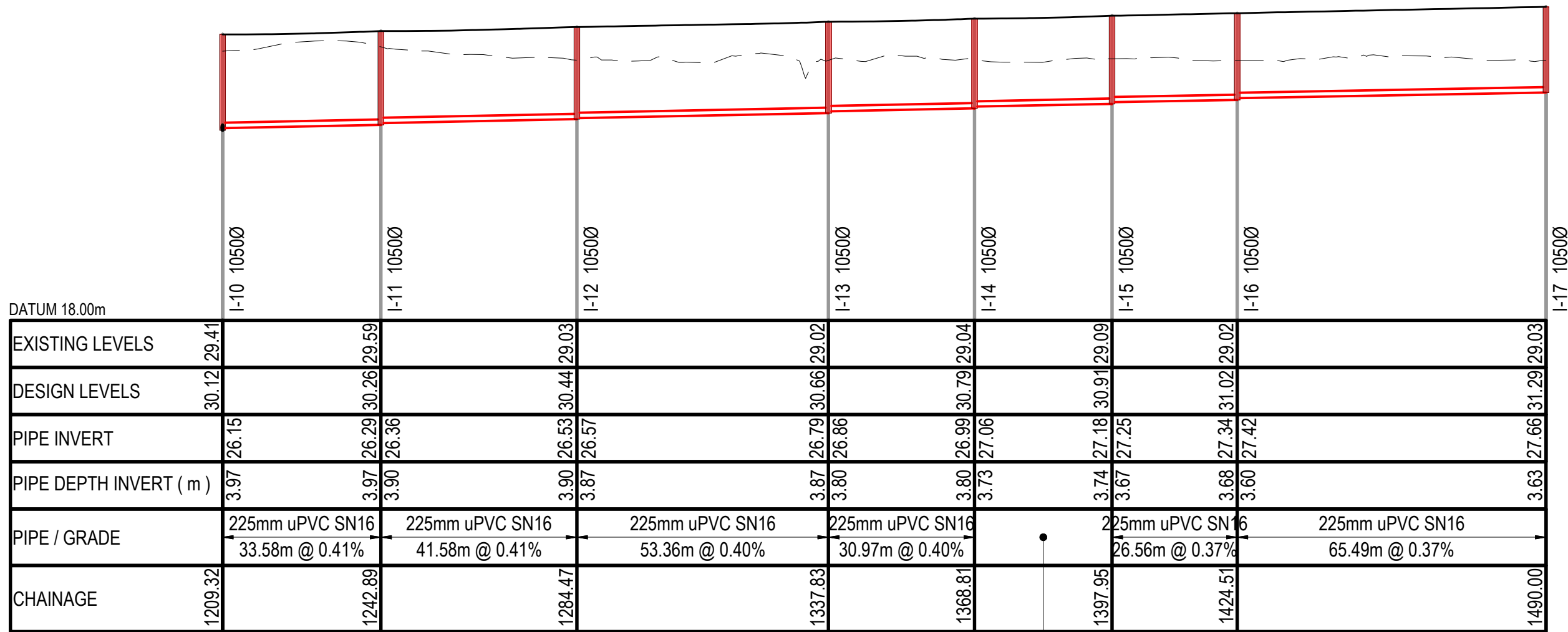
WASTEWATER LINE I SCALE: HORI 1:1000 VERT 1:200
