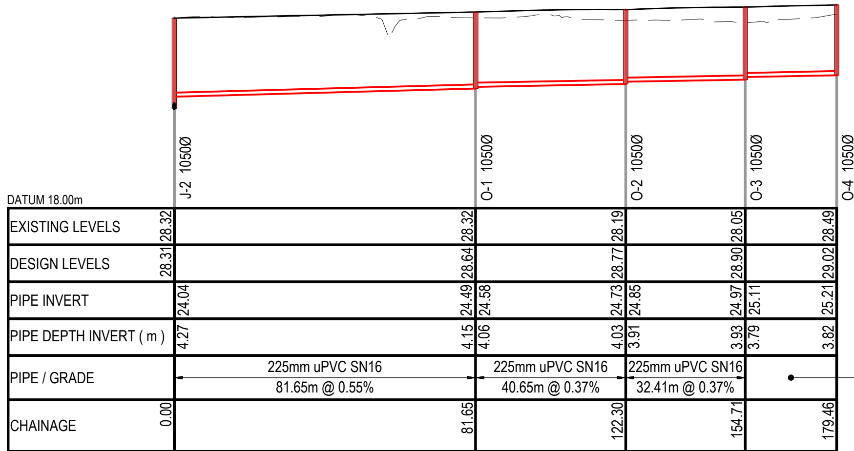
WASTEWATER LINE O SCALE: HORI 1:1000 VERT 1:200
