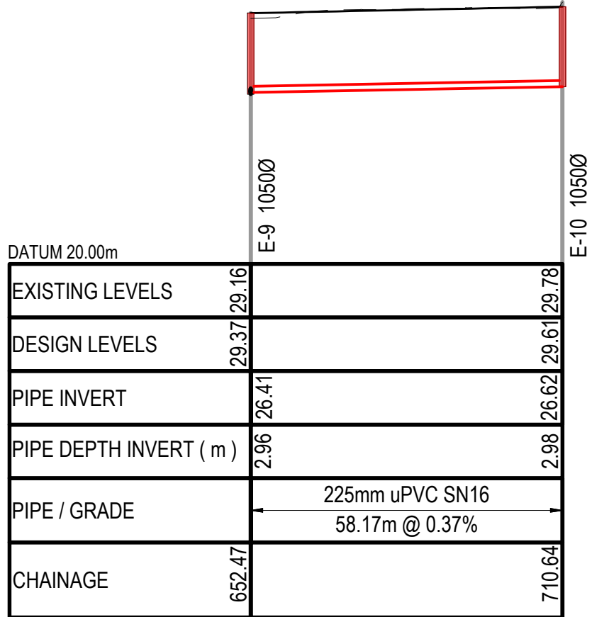
WASTEWATER LINE E SCALE: HORI 1:1000 VERT 1:200
