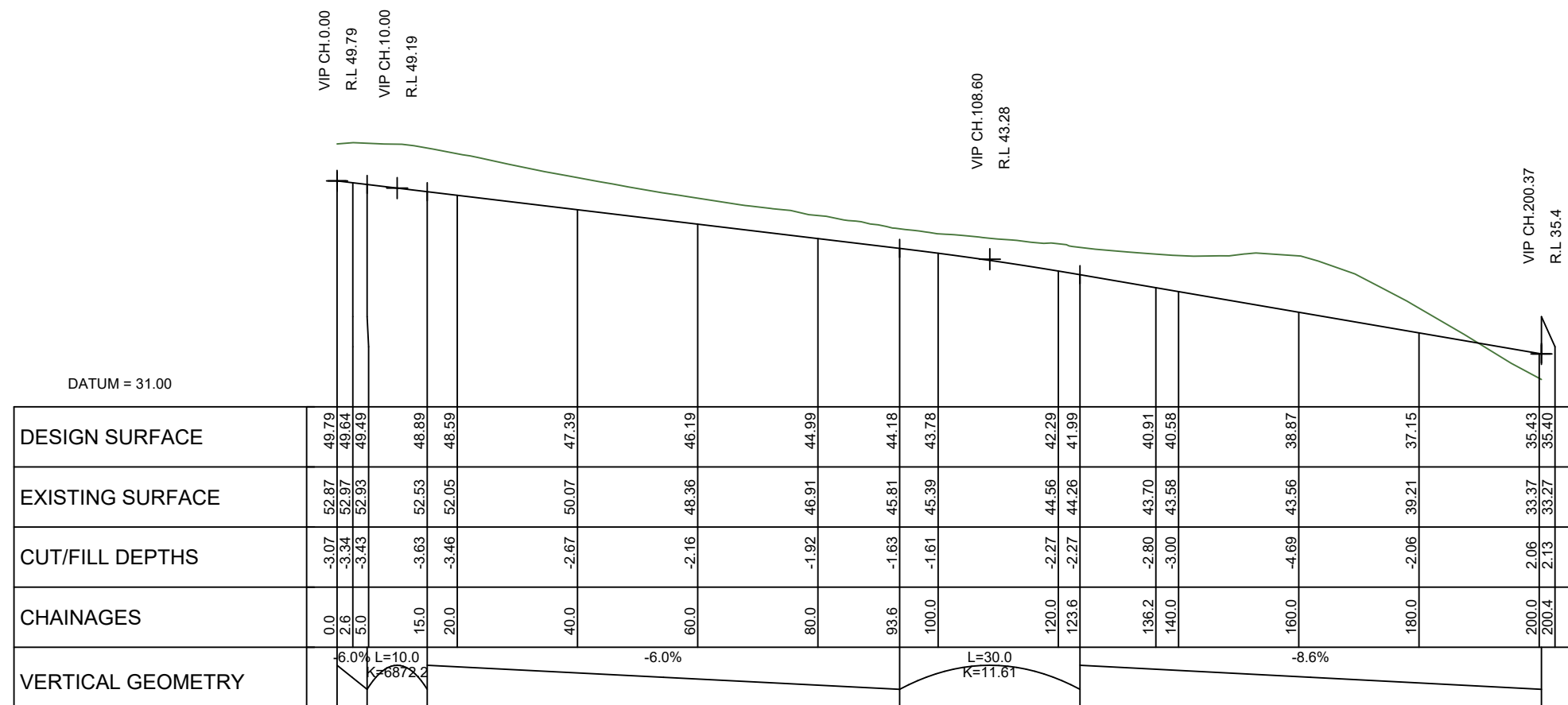
LONGITUDINAL SECTION JOAL 13
